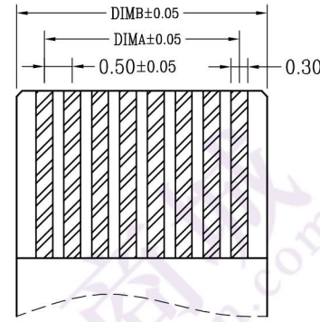
适用扁平线
